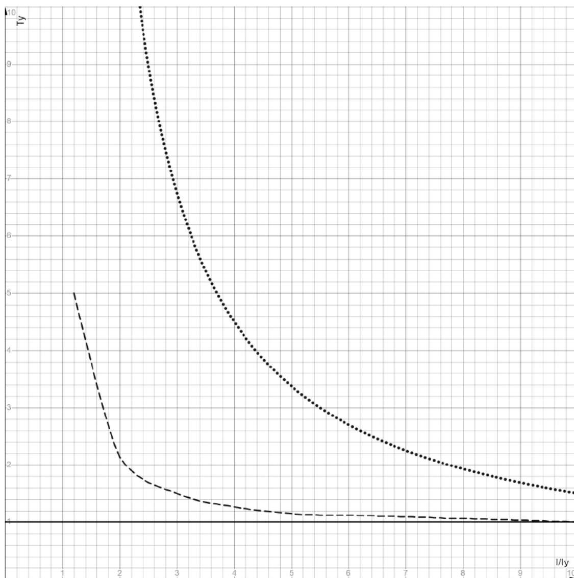
Рисунок Б.3 – Времятоковые характеристики тип “Независимая” (——), тип “Зависимая нормальная (нестандартизованная)” (— —) и “Зависимая крутая (РСТ-80АВ)” (— — —)
